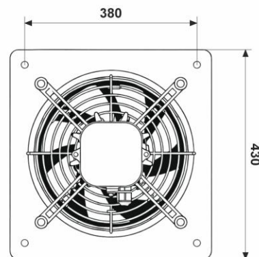
Dimensiones de montaje
