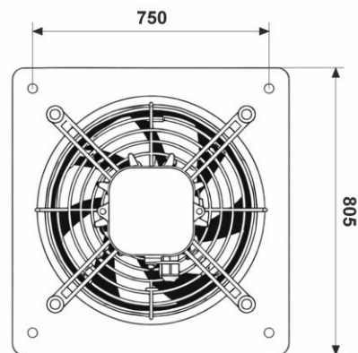
Dimensiones de montaje
