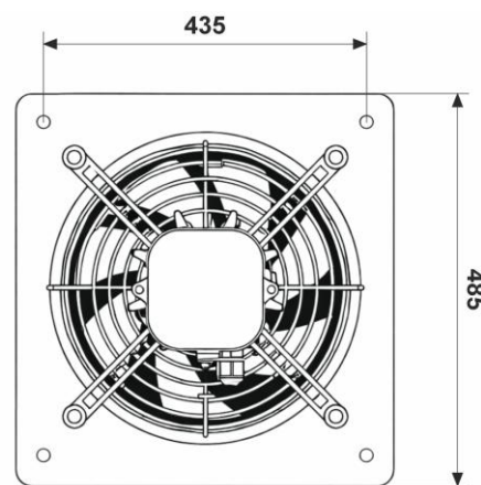
Dimensiones de montaje
